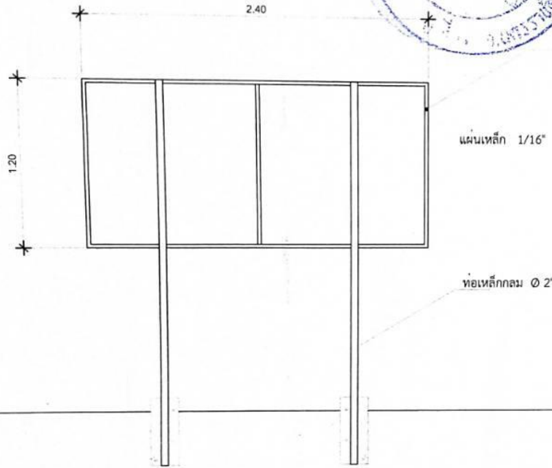
รูปด้านหลังป้ายโครงการ
