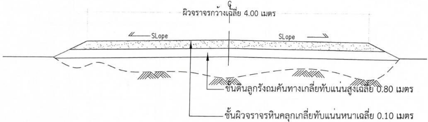
รูปตัดถนนแสดงการถมดินลูกรัง
