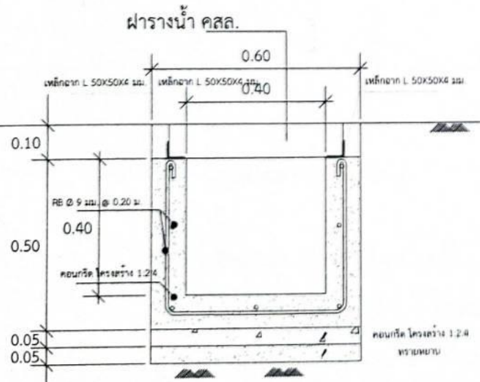
รูปตัด รางระบายน้ำ
