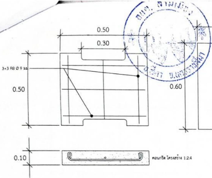
รูปขยาย ฝารางน้ำ คสล.
