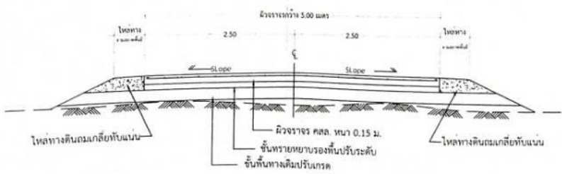
รูปตัดถนนรูปตัดแสดงโครงสร้างถนน SCALE no
