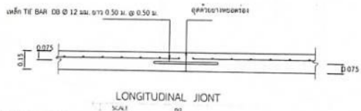
CONSTRUCTION JOINT (ทุกระยะ ไม่นเกิน 10 เมตร) SCALE no
